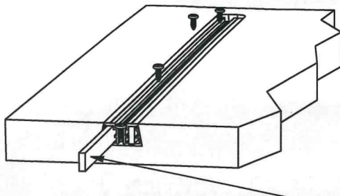
Variante 1: Verstärkung mit Stahlprofil Variant 1: Reinforcement with steel profile Variante 1 : renforcement avec profil acier Variante 1: refuerzo con perfil de acero Xx
