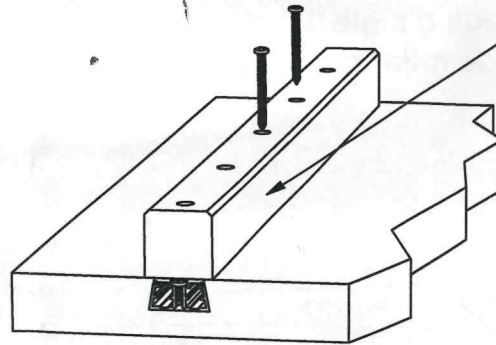
Variante 2: Verstärkung mit Holzleiste Variant 2: Reinforcement with wooden batten Variante 2 : renforcement avec latte en bois Variante 2: refuerzo con listón de madera Xx
