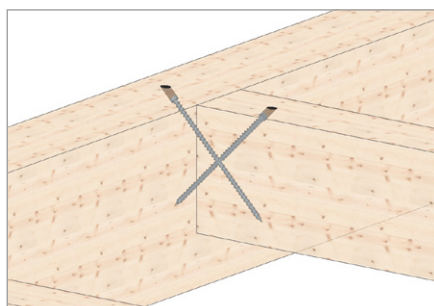
Stumpfe Querverbindung
