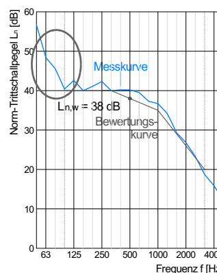
Abb. 39 Messwerte einer sichtbaren Massivholzdecke aus 148 mm Brettspertholz mit Deckenbeschwerung (100 mm Splitt, gefasst in Holzlatten). Die Bewertungskurve wird nach bestimmten Kriterien in die Messkurve verschoben. Der bewertete Trittschallpegel L_{n,w} wird dann bei 500 Hz abgelesen. Die hohen Werte im tieffrequenten Bereich werden dabei „übersehen“.
