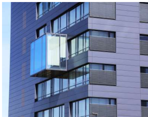
Abb. 58 Diese Fassade aus großformatigen Platten ist streng gegliedert. Dahinter verbirgt sich oftmals eine Unterkonstruktion aus Aluminium auf Punkthalterungen. Dieses System passt optimal zu Wänden aus Brettsperrholz.
