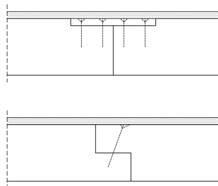
Abb. 36 Möglichkeiten für einen kraftschlüssigen Verbund von Brettsperrholzelementen. Oben Ausfaltung mit Streifen aus Holzwerkstoffen. Unten mit Wechselfalz.
