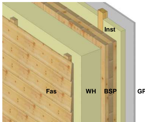
Abb. 53 Außenwände aus Brettsper Holz sind vom System her den Betonfertigteilen ähnlich. Drei Funktionsschichten prägen den Aufbau.
