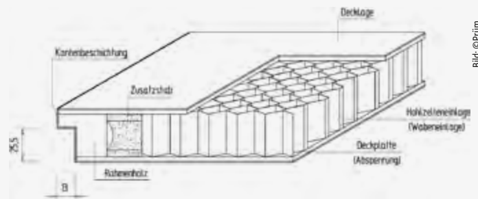
Innenleben einer Wabentür
