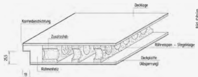
Innenleben einer Röhrenspanstreifentür
