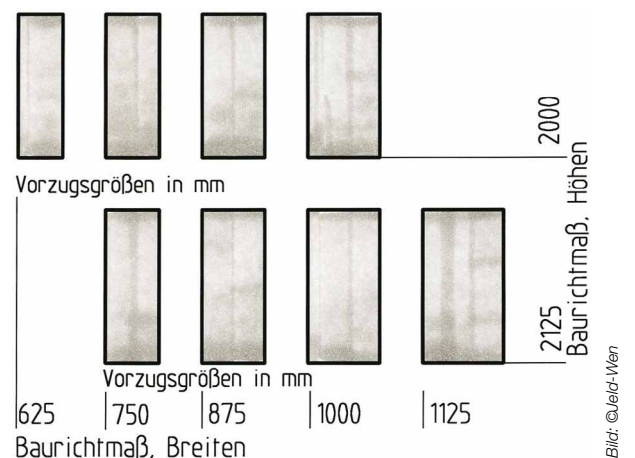
Rohbauöffnungen, die Vorzugsgrößen sind grau hinterlegt
