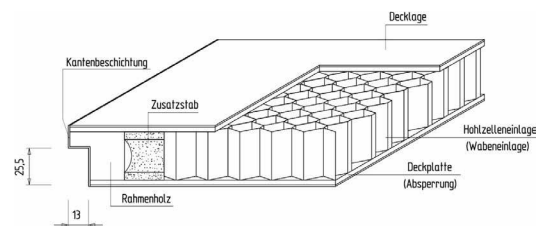
Innenleben einer Wabentür
