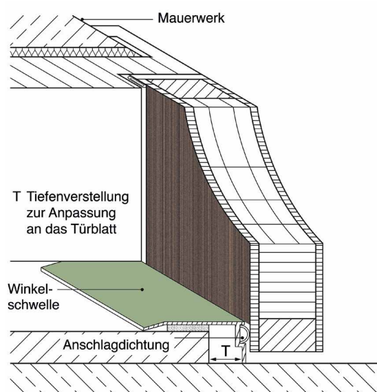
Anschlagsschwelle
