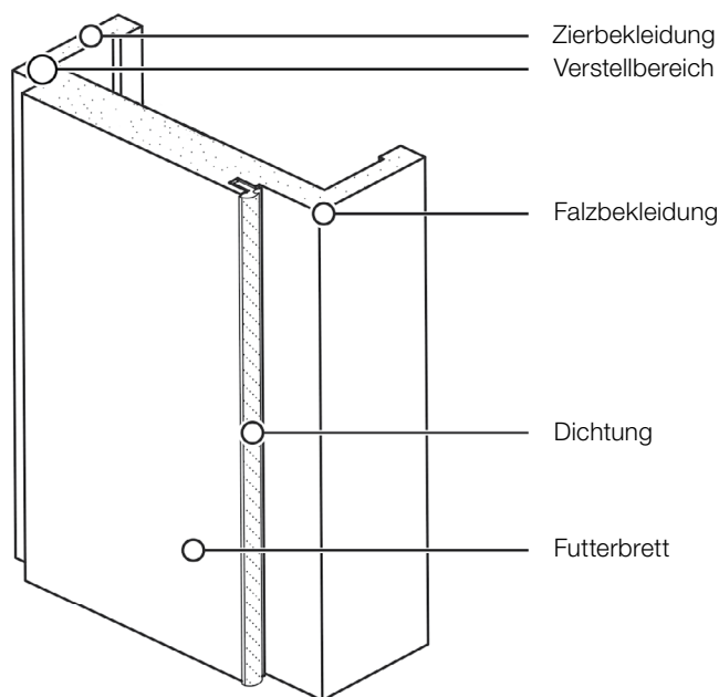
Konstruktionsdetails Umfassungszarge
