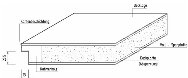
Innenleben einer Vollspantür
