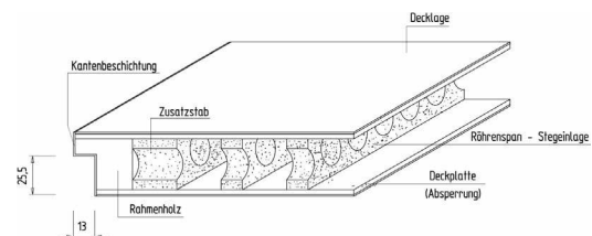
Innenleben einer Röhrenspanstreifentür
