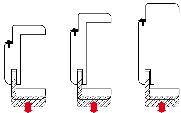
Verstellbereich Umfassungszarge
