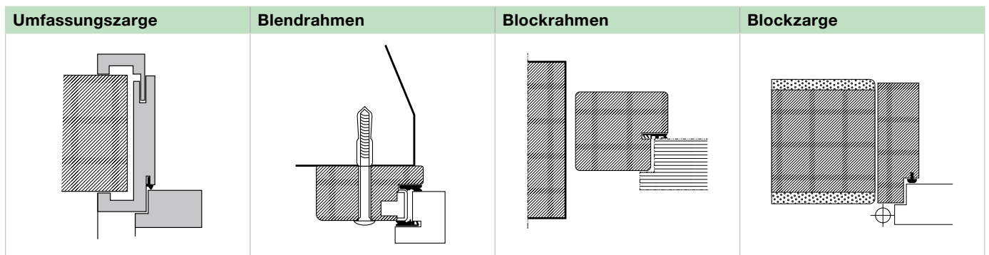
Konstruktionsarten Türrahmen und Türzargen
