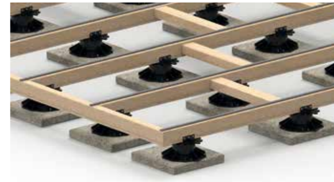
Zur Absicherung der Windlasten müssen z. B. bei Dachterrassen die Verstellfüße an der Unterkonstruktion sowie auf den Betonplatten befestigt werden.
