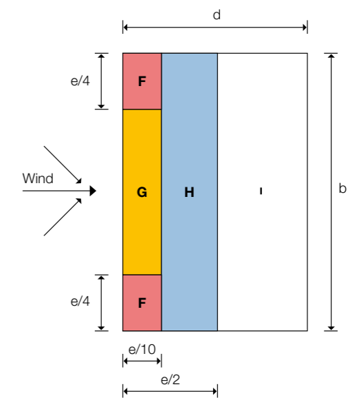
Einteilung der Flächen ( e = b oder 2h )
